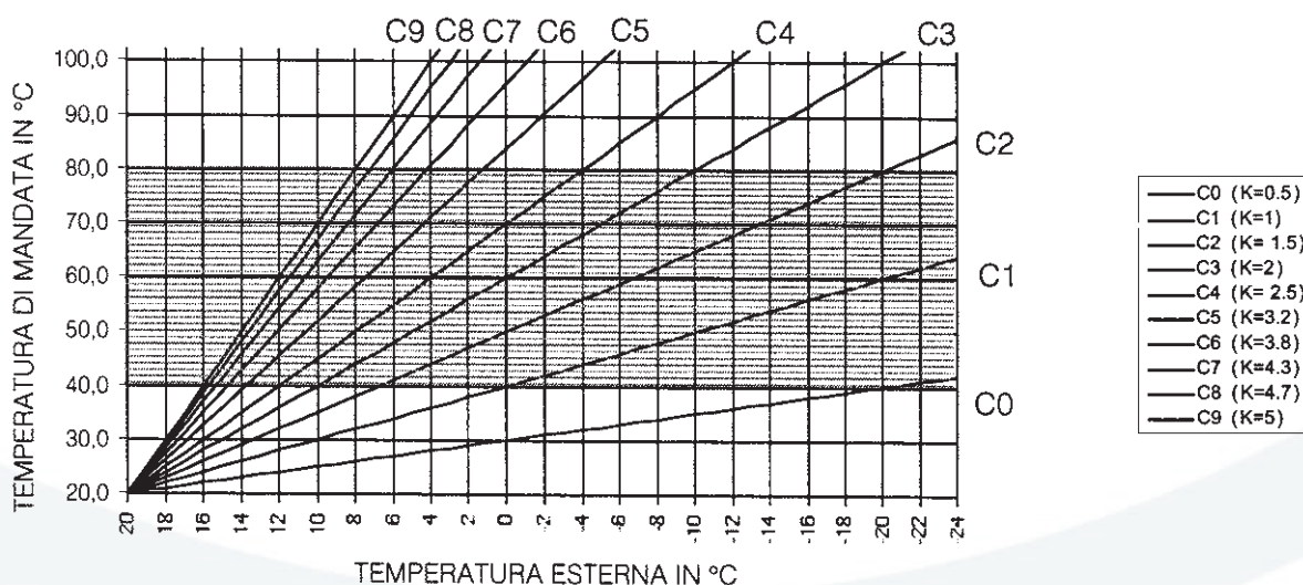
TEMPERATURA MANDATA DI CALDAIA/TEMPERATURA ESTERNA (BANCO 0)
