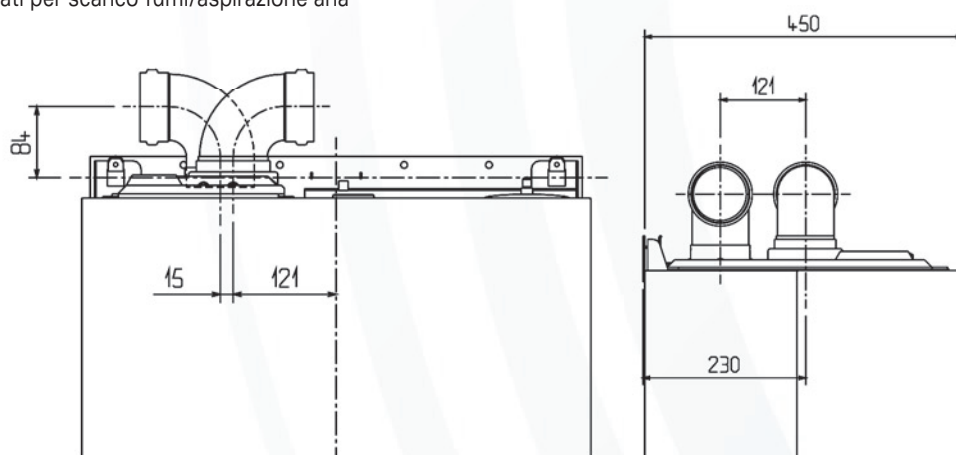
Condotti sdoppiati per scarico fumi/aspirazione aria
