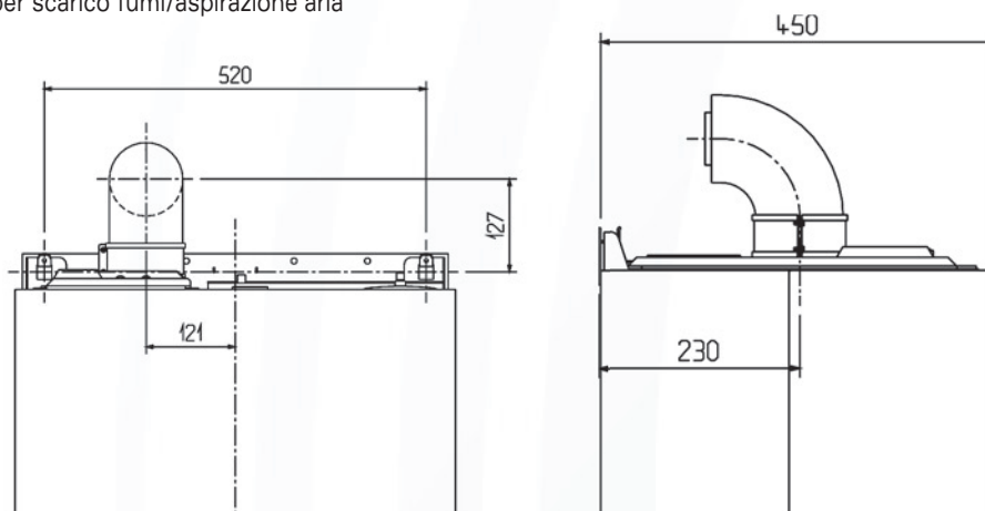
Condotto concentrico per scarico fumi/aspirazione aria
